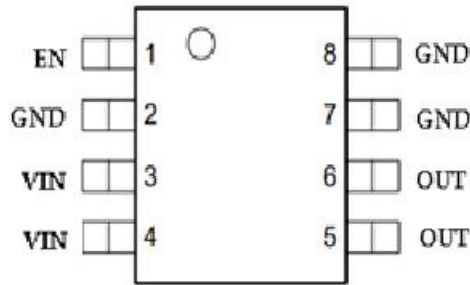
图3-1 BSS6050H管脚图
