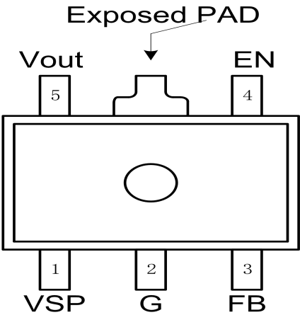
图 2 引脚定义图
